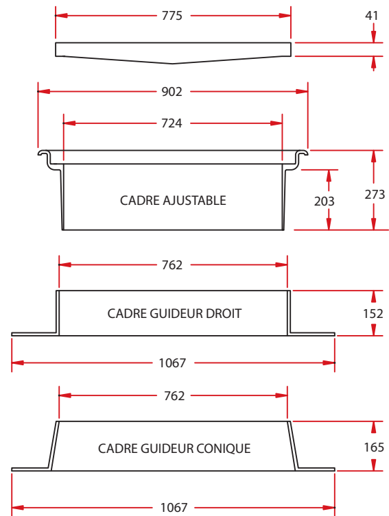
CADRE et COUVERCLE CT-6A
